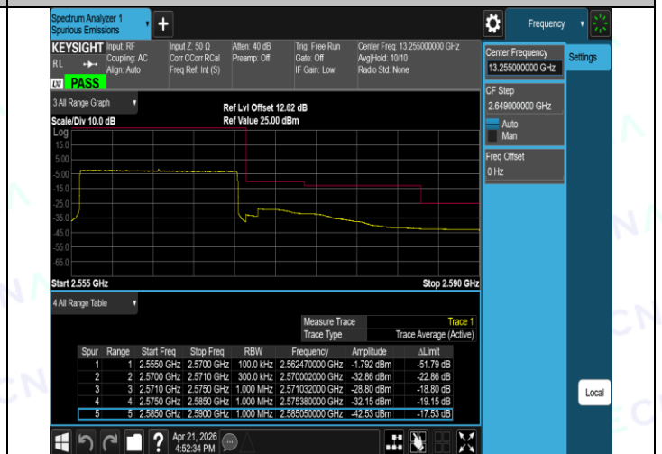
Band7-20MHz-QPSK-20850-1RB#99-PASS
