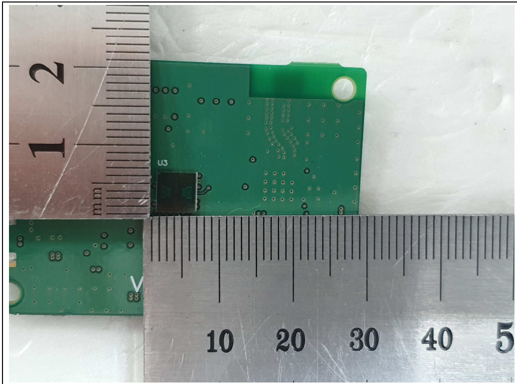
<Rader Module>
