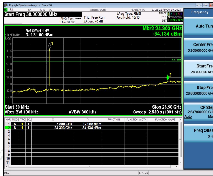
Ant1_5847_0~Reference
