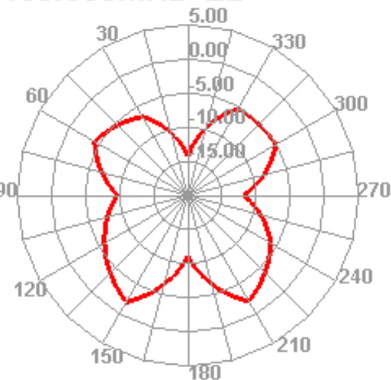
2400.000MHz E2
