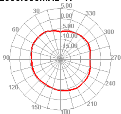
2500.000MHz H
