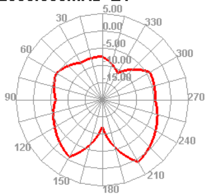
2500.000MHz E1
