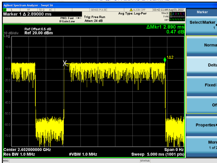
\pi/4 -DQPSK 2DH5 2402MHz
