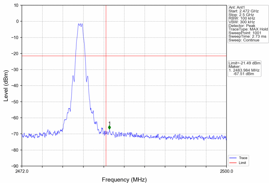
HCH_2480MHz_Ant1_NTNV
