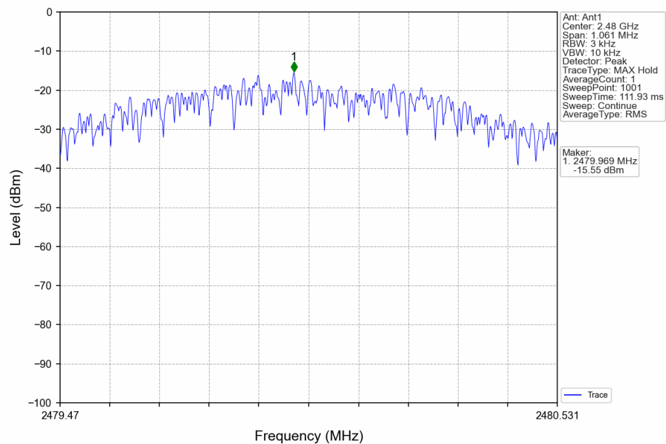
HCH_2480MHz_Ant1_NTNV
