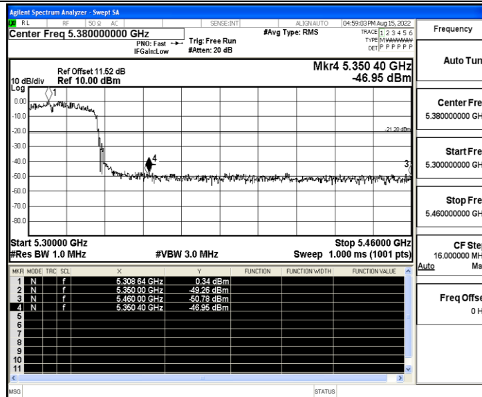
11AC80SISO_Ant0_Low_5290_AV
