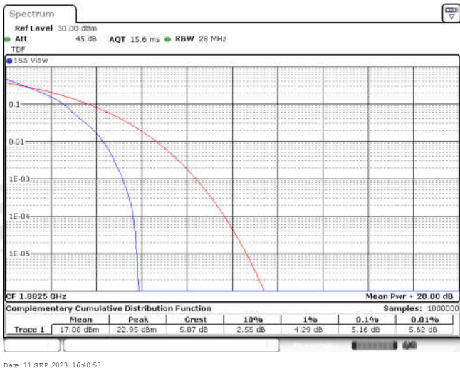
Band25-5MHz-QPSK-26365-25RB#0
