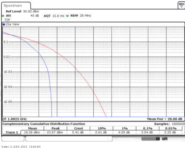
Band25-1.4MHz-QPSK-26365-6RB#0
