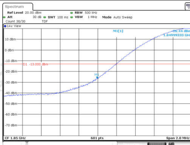
Band25-20MHz-QPSK-26140-1RB#0
