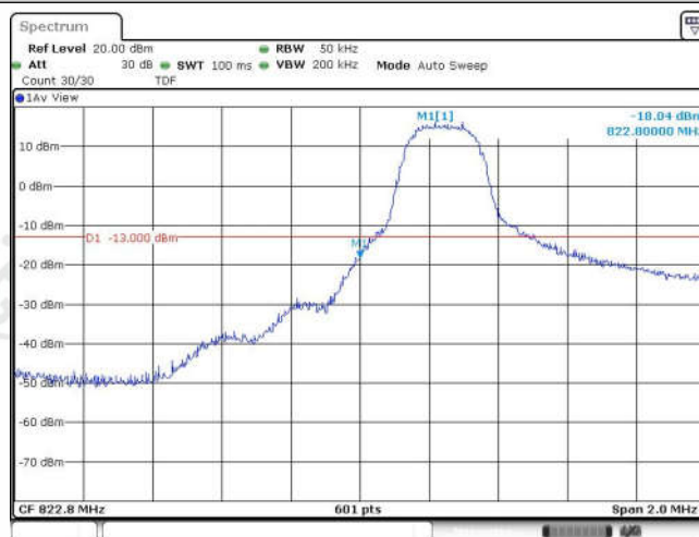
Band26-3MHz-QPSK-26793-1RB#0
