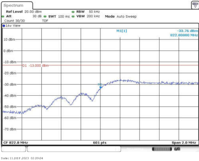
Band26-3MHz-QPSK-26793-15RB#0
