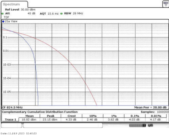
Band26-3MHz-QPSK-26793-15RB#0
