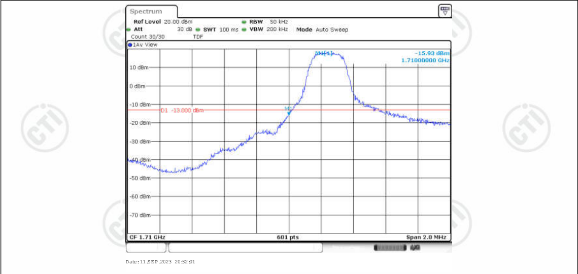
Band4-3MHz-QPSK-19965-1RB#14
