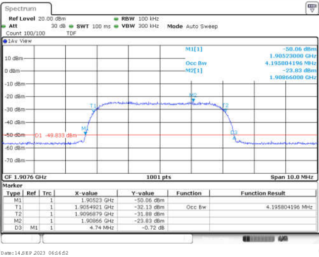
Band2-9538-5
