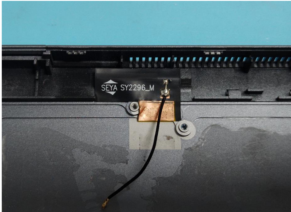
Wi-Fi ANT1
