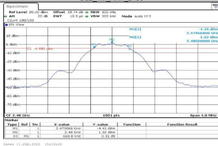
BLE 1M Ant1_2480
