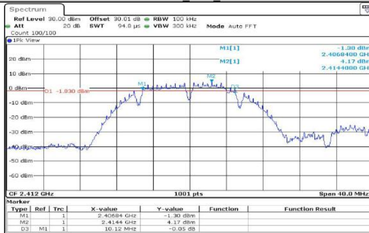
11B-CDD_Ant1_2412
