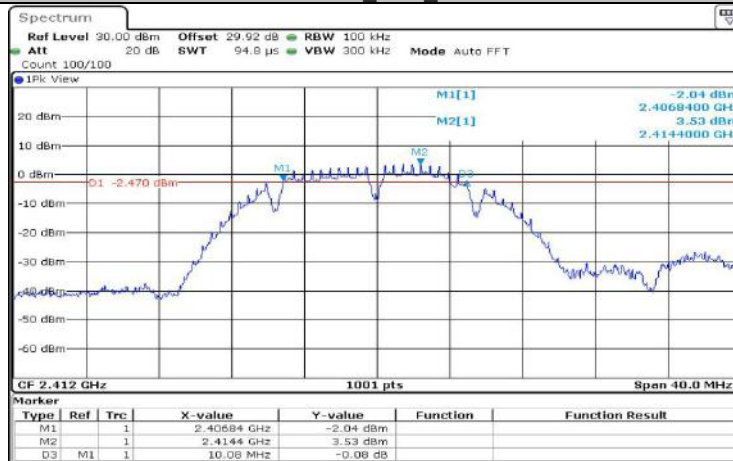
11B-CDD_Ant2_2412
