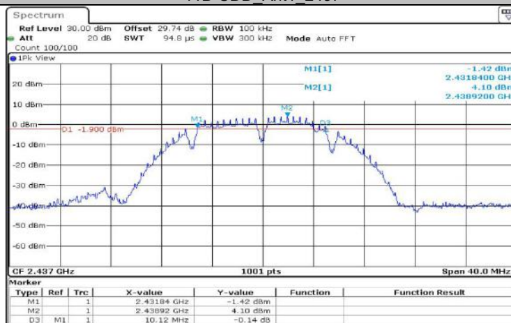
11B-CDD_Ant1_2437
