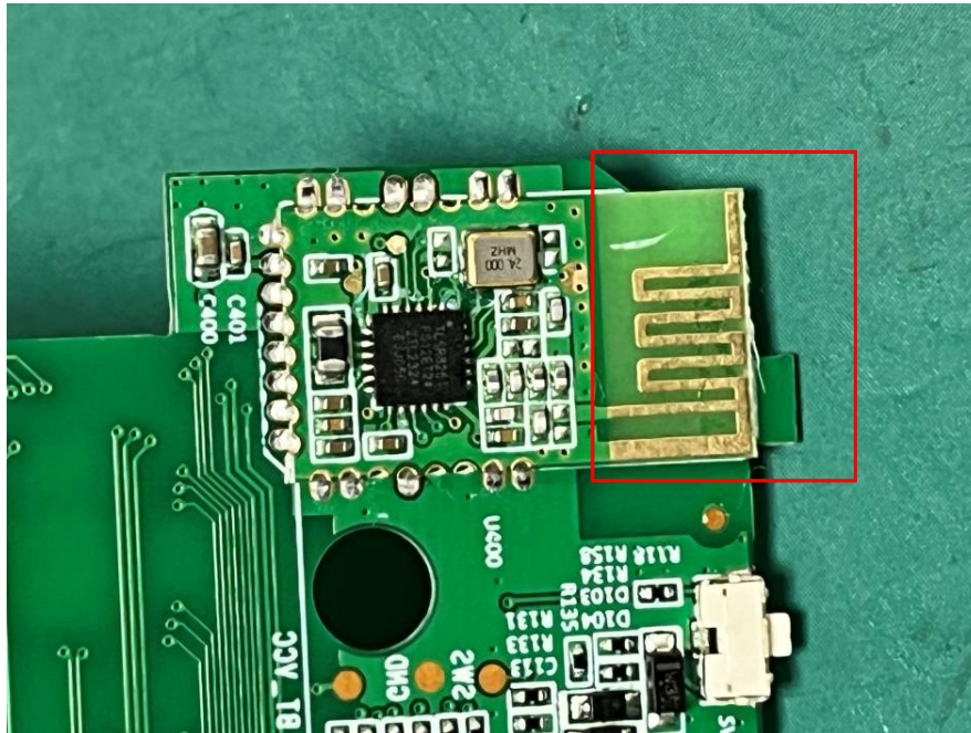
BLE ANT
