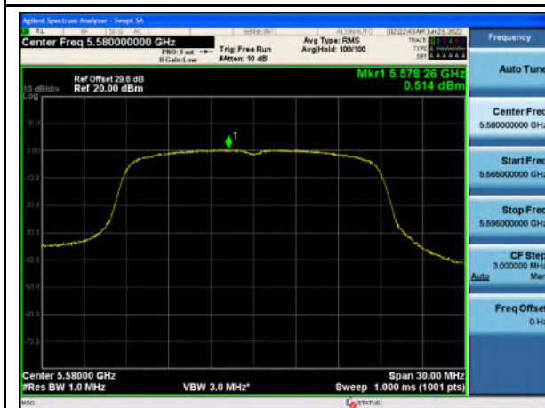
PSD_U-NII-2C_802.11n_5580
