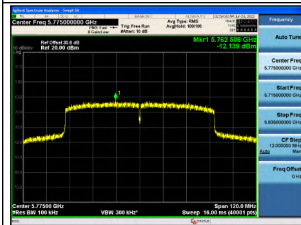
PSD_U-NII-3_802.11ac80_5775
