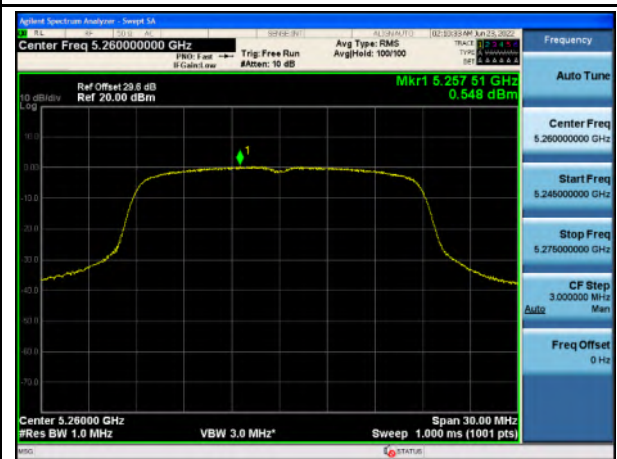
PSD_U-NII-2A_802.11n_5260
