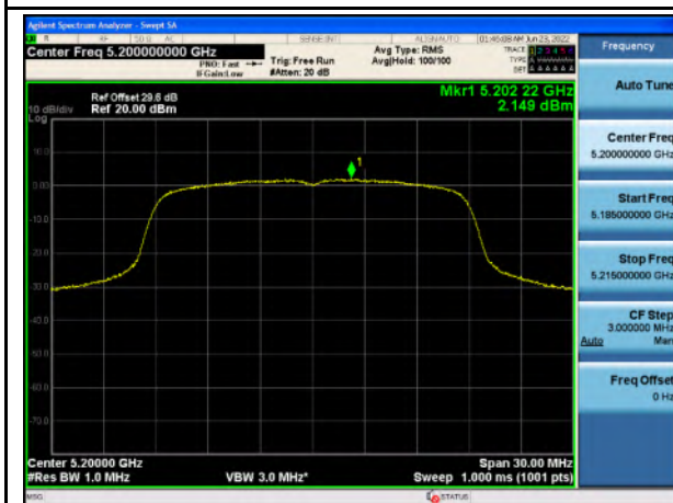
PSD_U-NII-1_802.11n_5200
