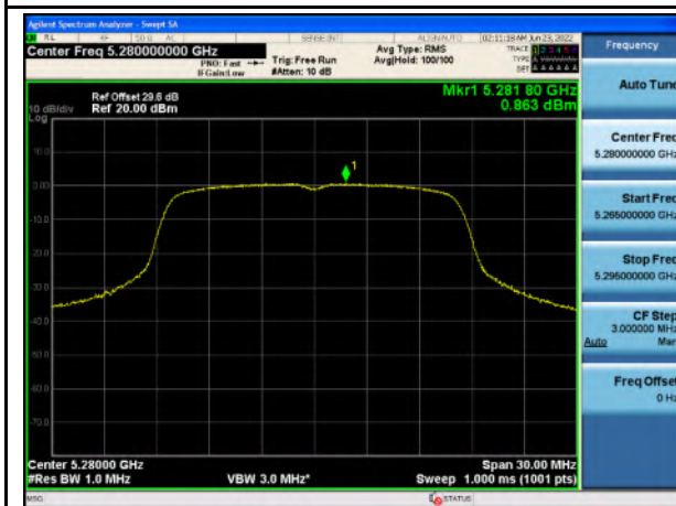
PSD_U-NII-2A_802.11n_5280
