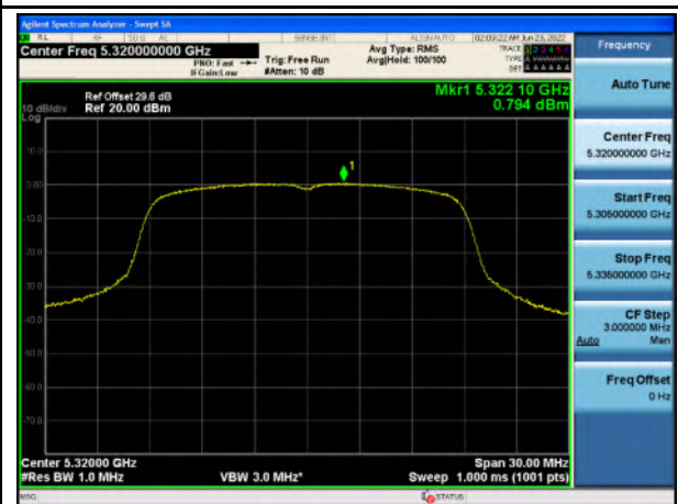
PSD_U-NII-2A_802.11n_5320
