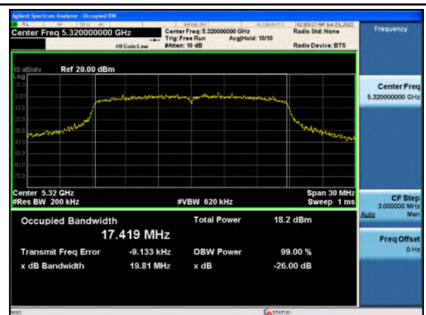
26 dB & 99% BW_U-NII-2A_802.11n_5320
