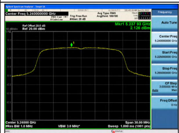
PSD_U-NII-1_802.11n_5240
