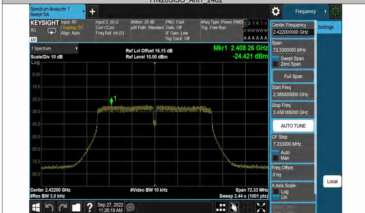
11N40SISO Ant1 2422
