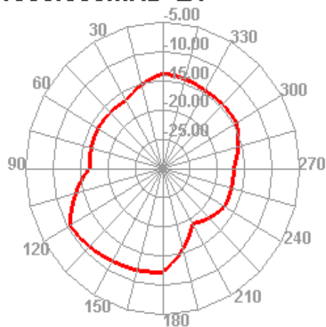
1000.000MHz E1
