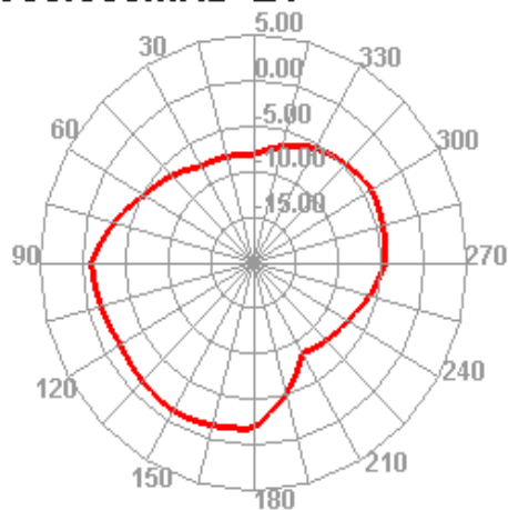
930.000MHz E1
