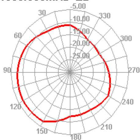
1000.000MHz E2
