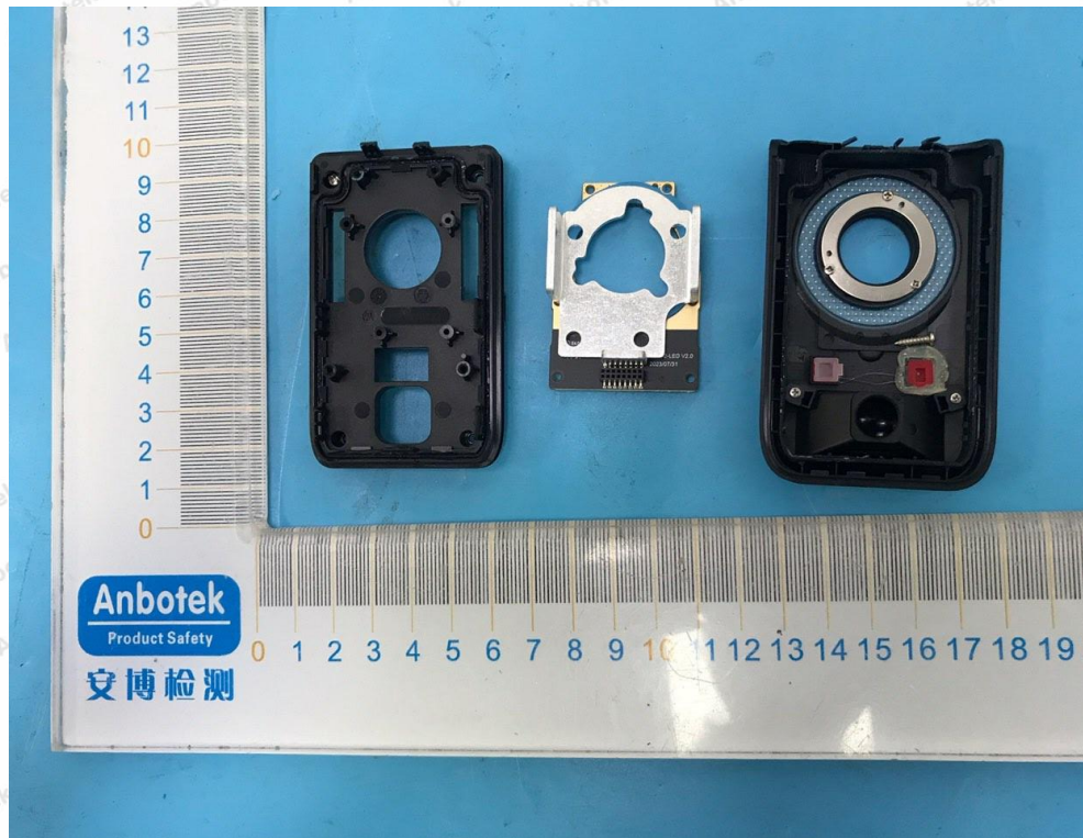
RX ANT--RADAR
