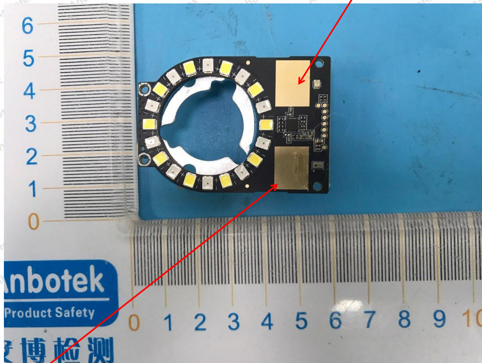
TX ANT--RADAR
