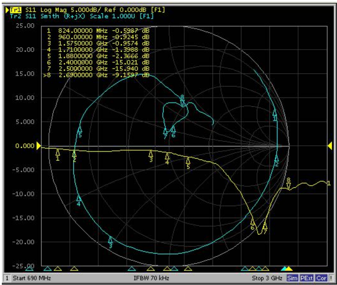
S11 (图 1)
