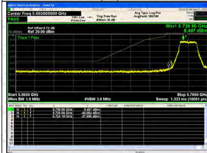
802.11(n40)-5755
