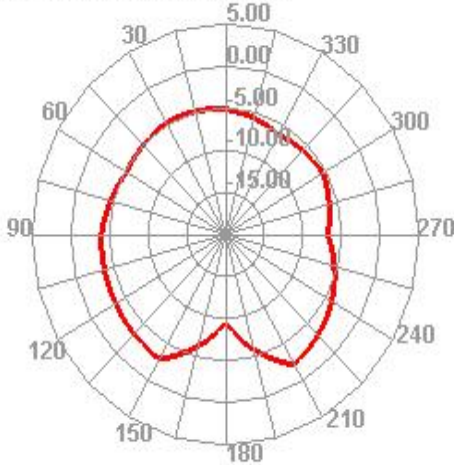
2420.000MHz E2
