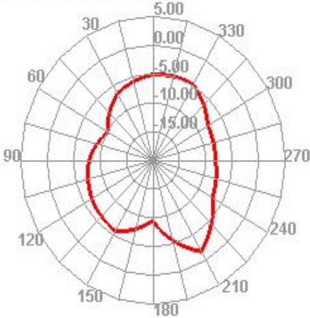
2420.000MHz E1
