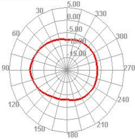
2420.000MHz H
