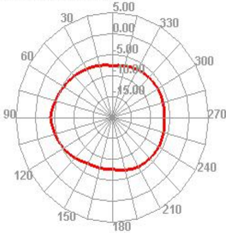
2430.000MHz H
