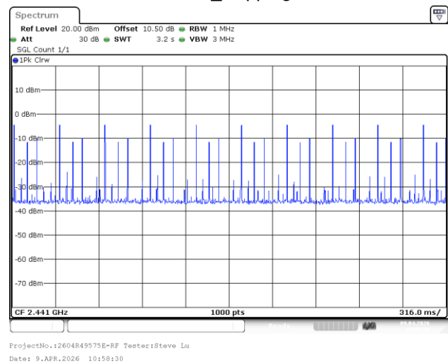
2DH5_Hopping
