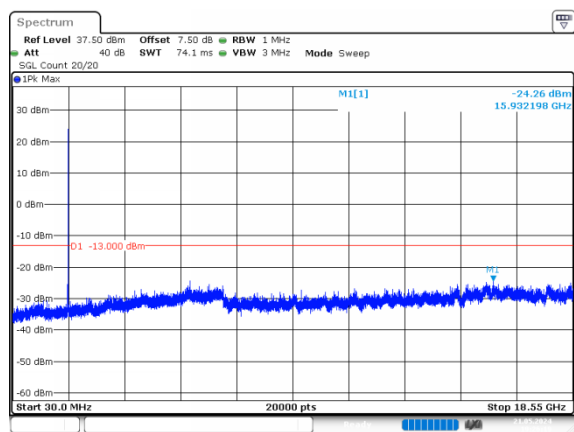
10MHz_Low_QPSK_1@0
