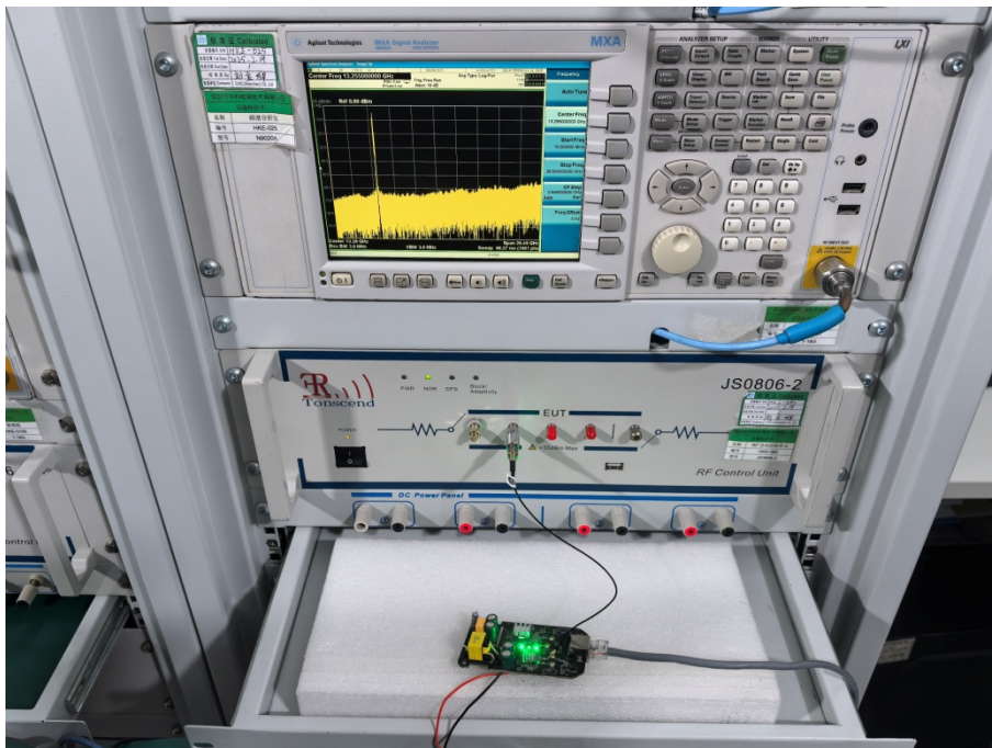
5.8G WIFI ANT1
