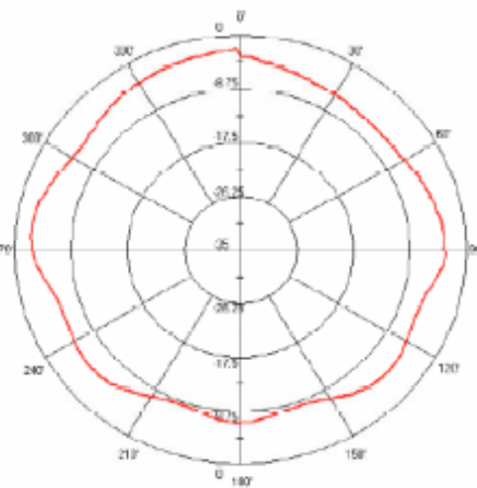
2.4 GHz H-Plane Horizontal
