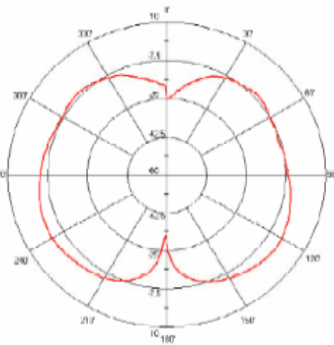
2.4 GHz H-Plane Horizontal
