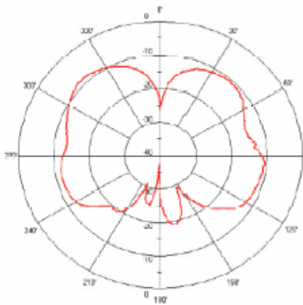
2.4 GHz H-Plane Vertical
