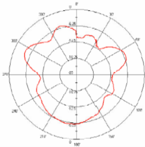
2.4 GHz H-Plane Vertical
