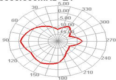
5000.000MHz E1
