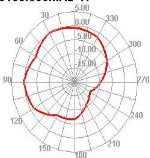
5100.000MHz H
