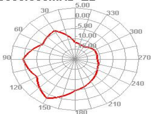
5000.000MHz E2
