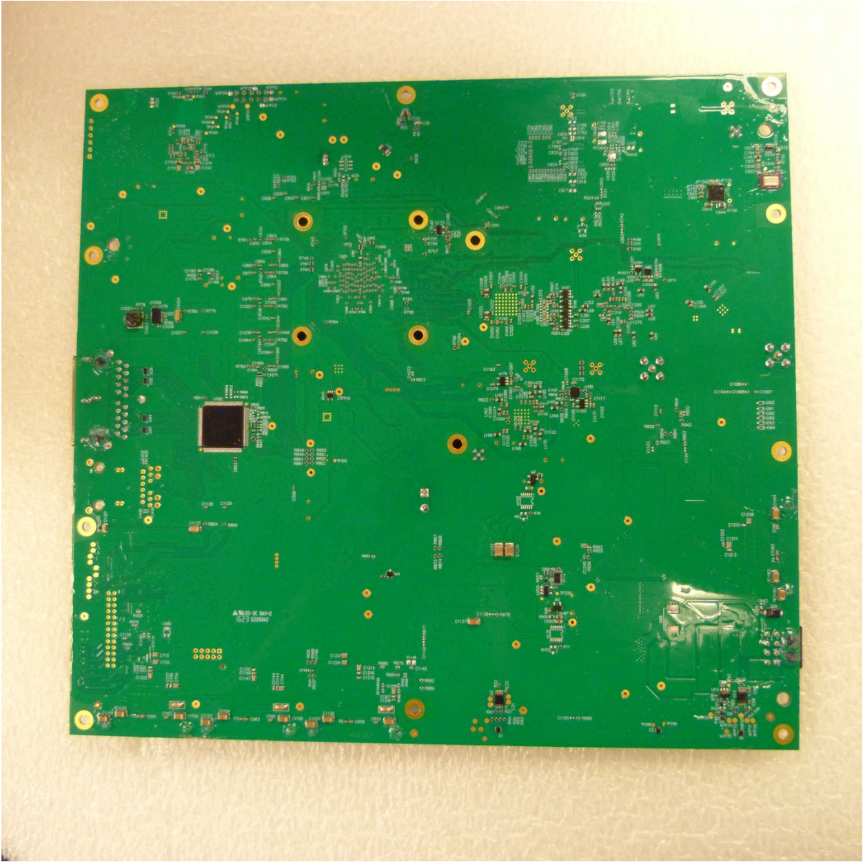
ACU Back
