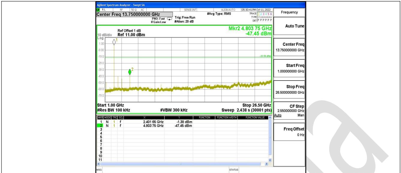
DH1_Ant1_2402_1000~26500
