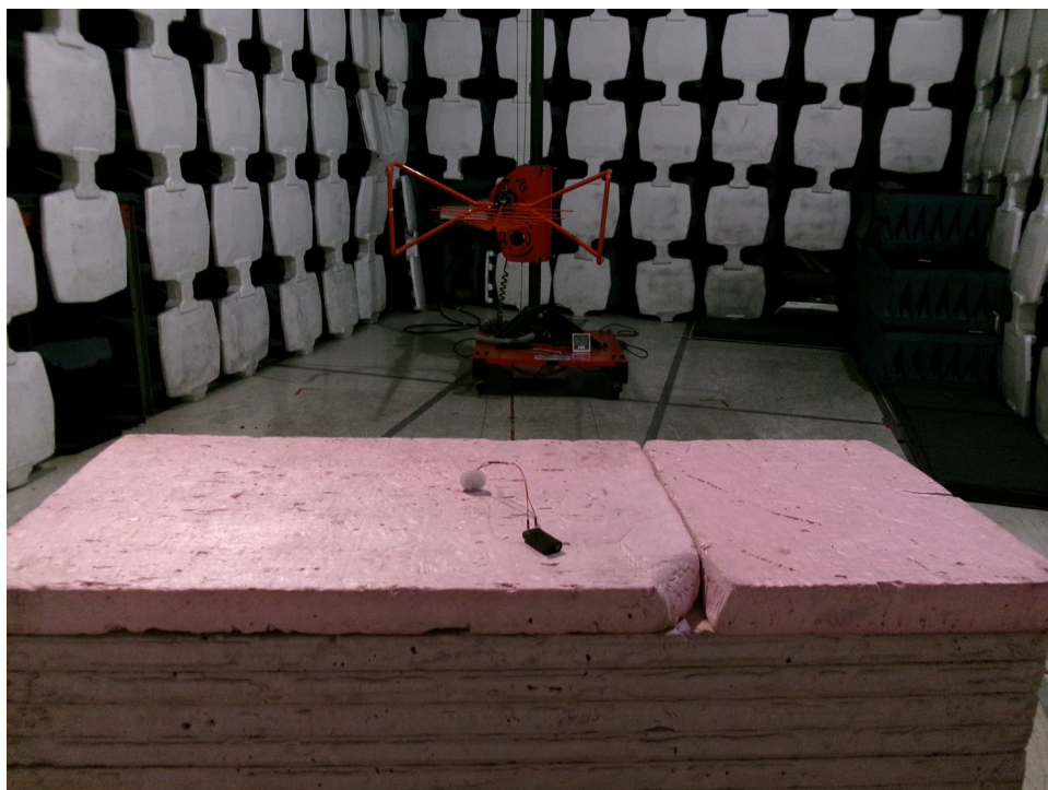
30-1000MHz
