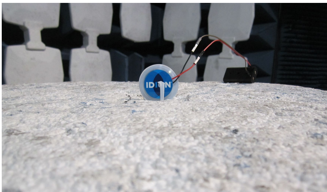
EUT – Y-Axis
