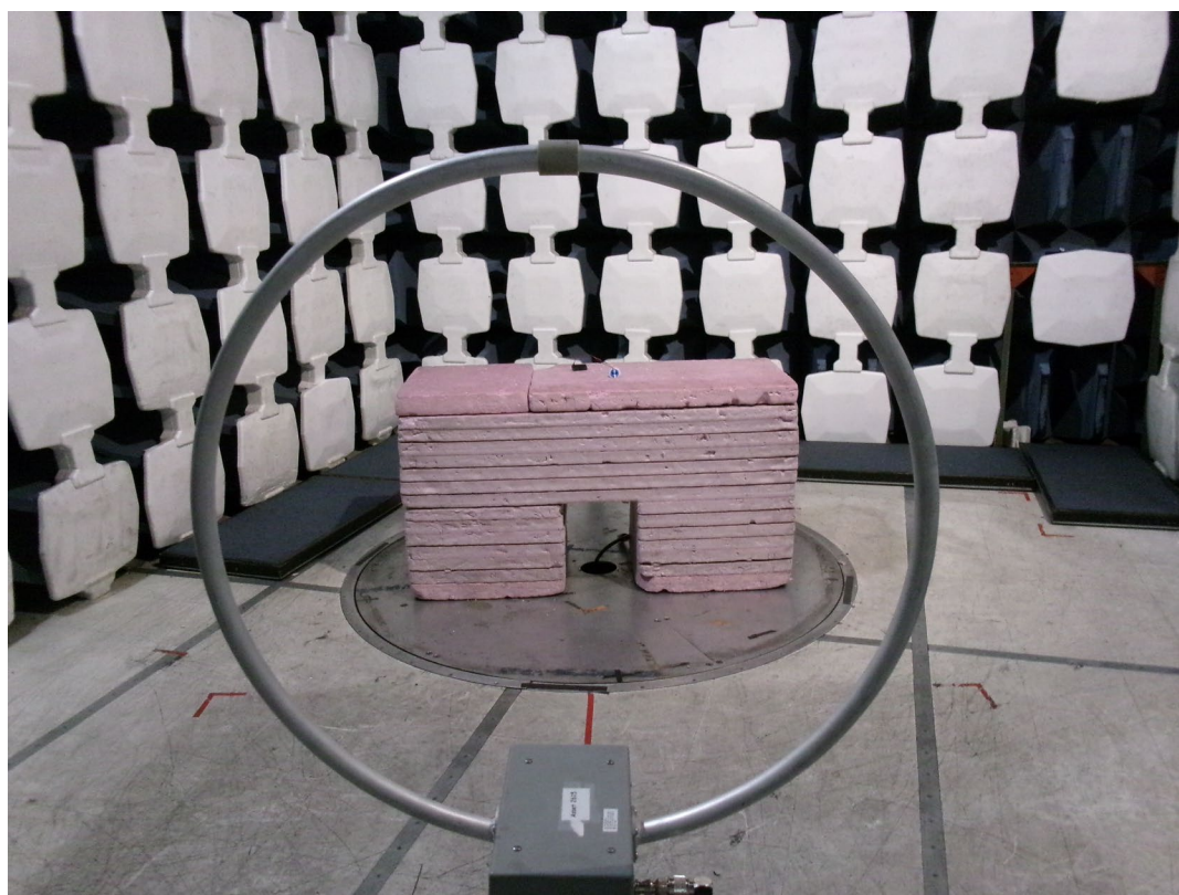
9kHz – 30MHz
