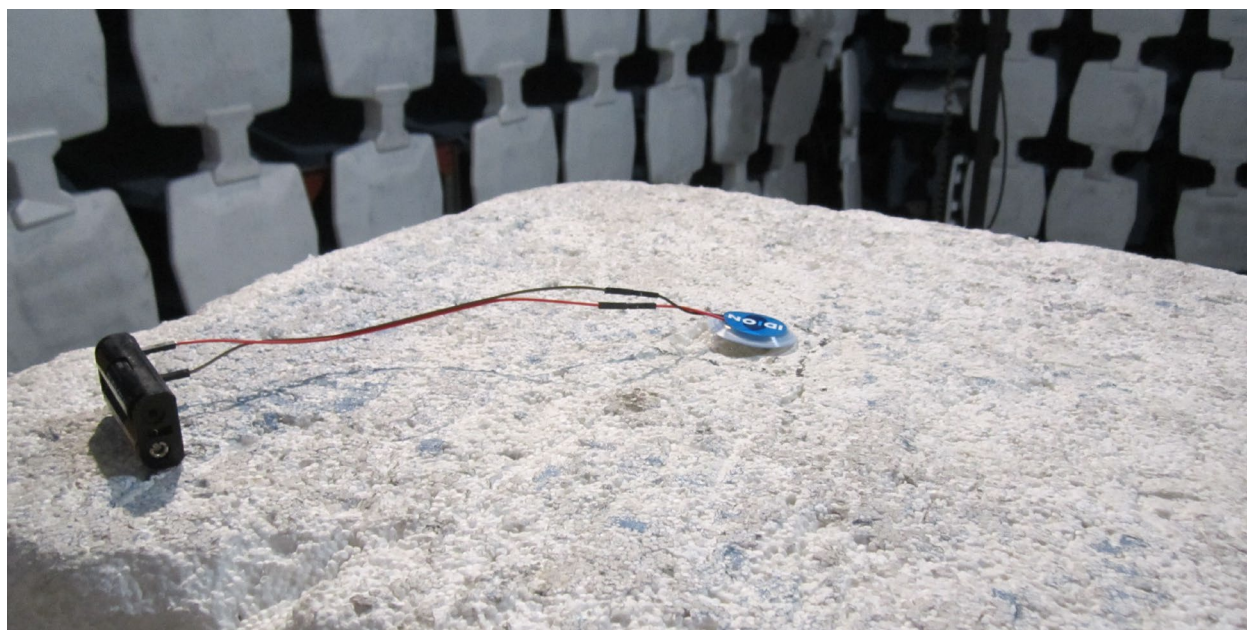
EUT – X-Axis
