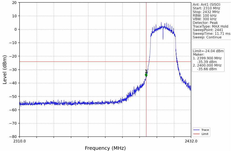
802.11n(HT20)_LCH_2412MHz_Ant1 (SISO)_NTNV
