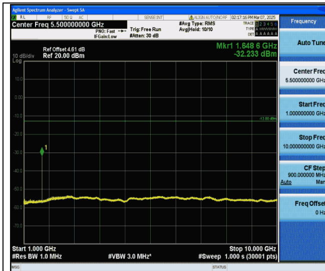
GPRS850-128-5-1000~10000MHz-PASS
