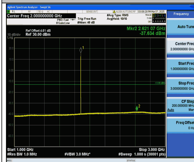
EGPRS1900-661-2-1000~3000MHz-PASS
