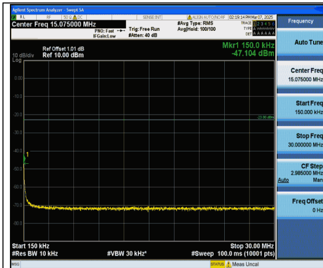
GPRS850-251-5-0.15~30MHz-PASS
