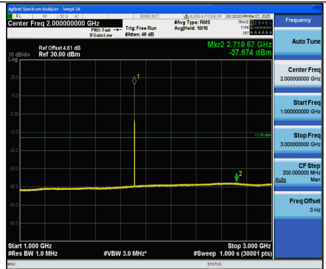
EGPRS1900-810-2-1000~3000MHz-PASS
