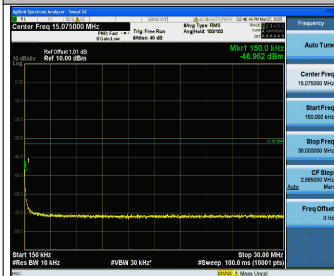
GPRS1900-512-0-0.15~30MHz-PASS
