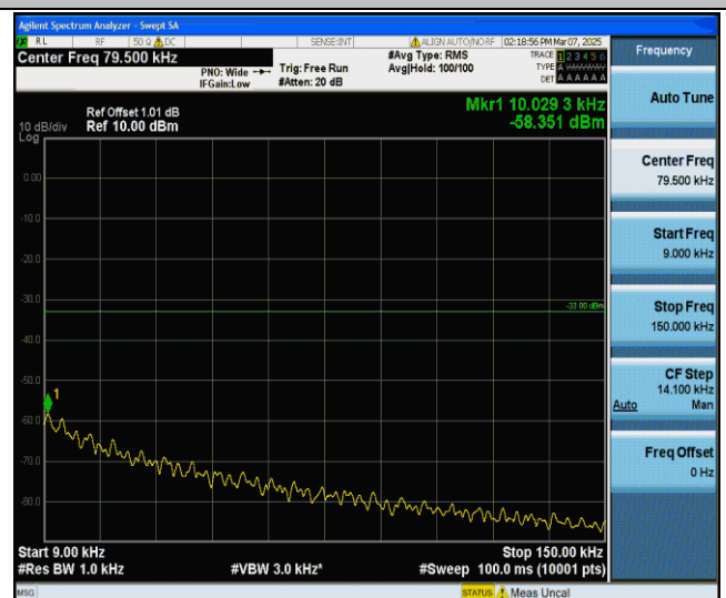
GPRS850-251-5-0.009~0.15MHz-PASS
