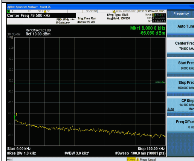
EGPRS850-190-8-0.009~0.15MHz-PASS
