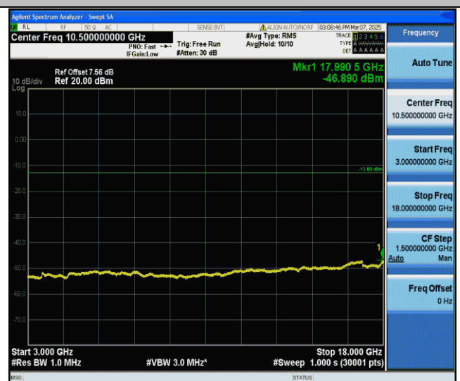
EGPRS1900-661-2-3000~18000MHz-PASS
