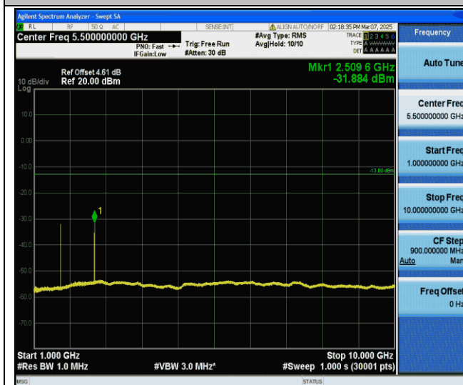
GPRS850-190-5-1000~10000MHz-PASS
