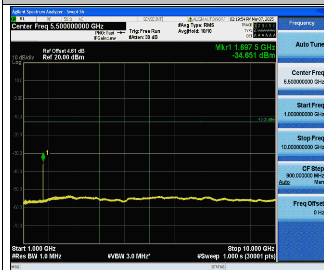
GPRS850-251-5-1000~10000MHz-PASS
