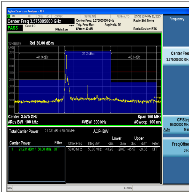
NTVN-n48-PC3-30-50-L-CP-QPSK-Inner_1RB_Left-PASS
