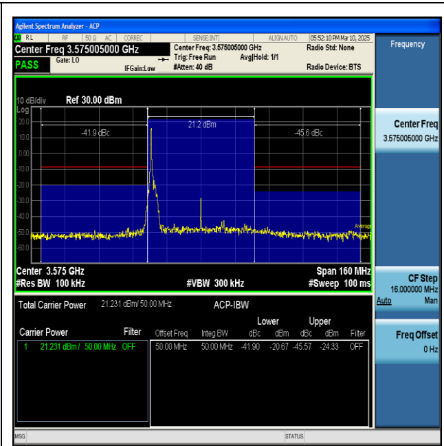
NTVN-n48-PC3-30-50-L-CP-QPSK-Inner_1RB_Left-PASS
