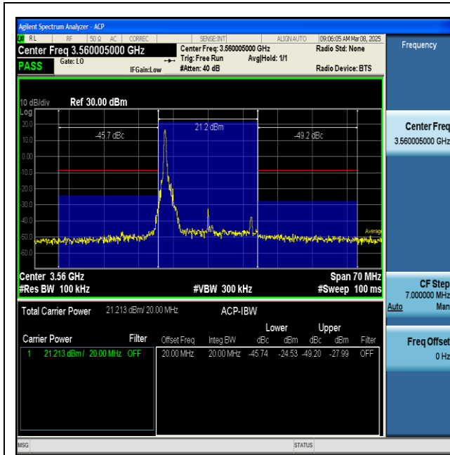
NTVN-n48-PC3-30-20-L-CP-QPSK-Inner_1RB_Left-PASS
