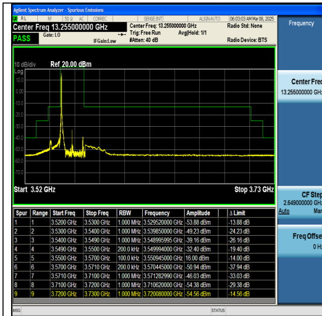
NTNV-n48-PC3-30-20-L-DFT-BPSK-Edge_1RB_Left-PASS
