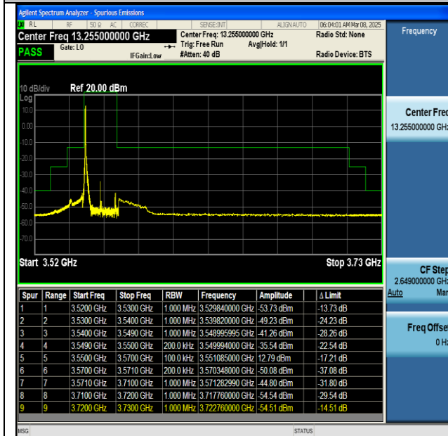
NTNV-n48-PC3-30-20-L-CP-QPSK-Edge_1RB_Left-PASS
