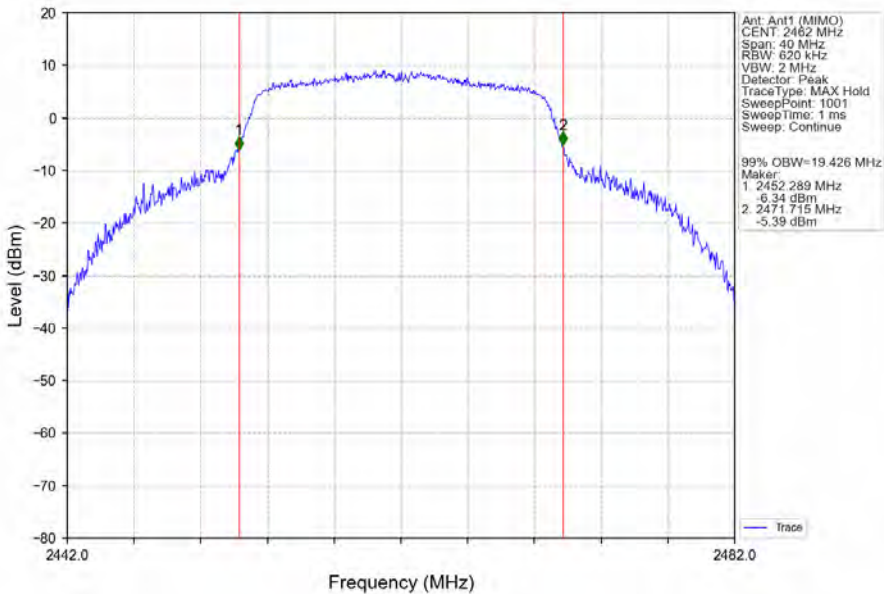
802.11n(HT20)_HCH_2462MHz_Ant1 (MIMO)_NTNV
