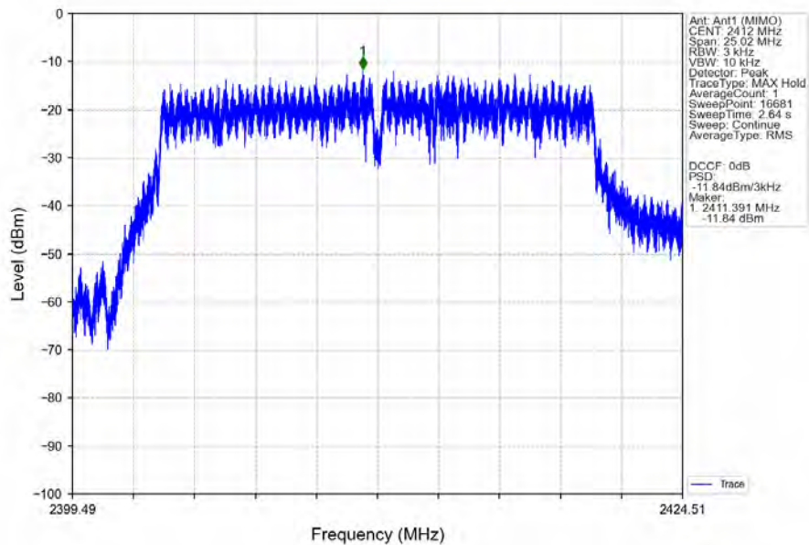
802.11n(HT20)_LCH_2412MHz_Ant1 (MIMO)_NTNV
