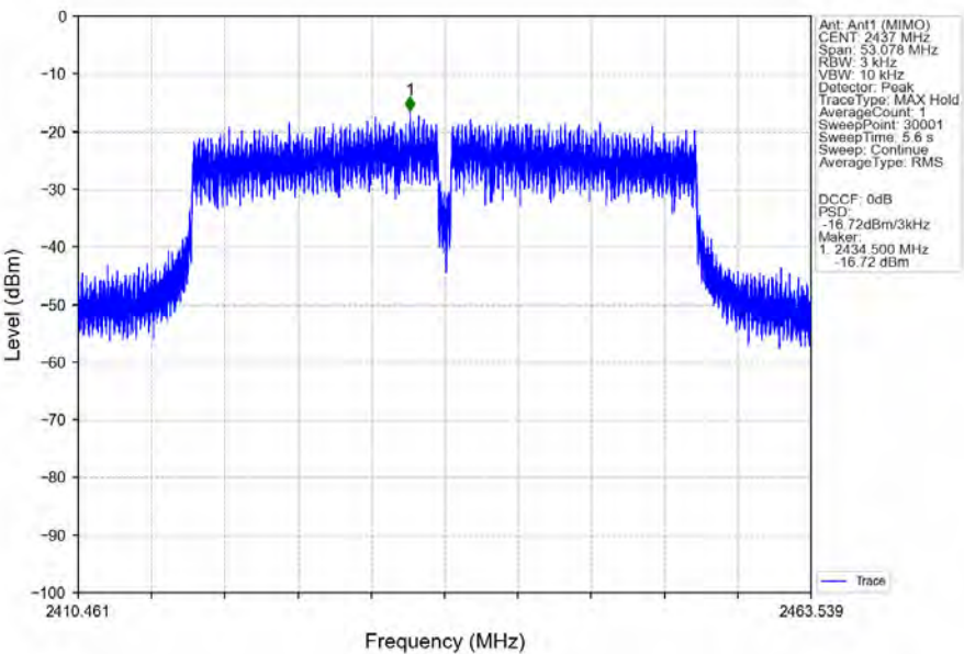
802.11n(HT40)_MCH_2437MHz_Ant1 (MIMO)_NTNV
