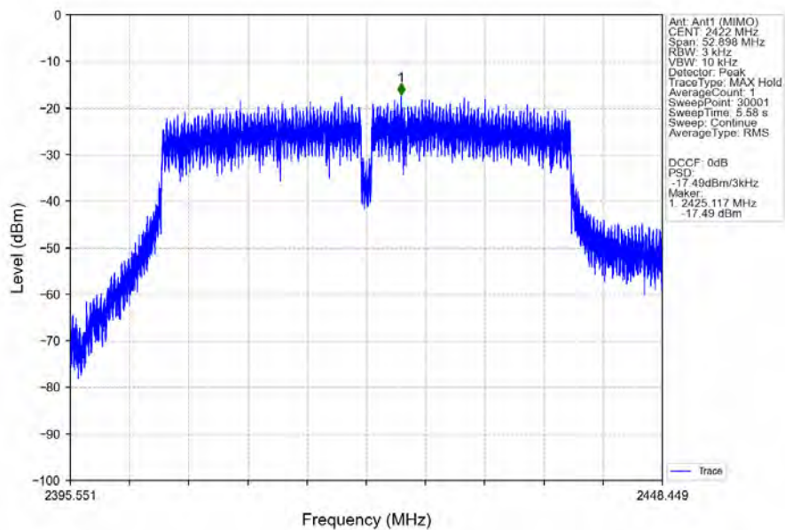
802.11n(HT40)_LCH_2422MHz_Ant1 (MIMO)_NTNV
