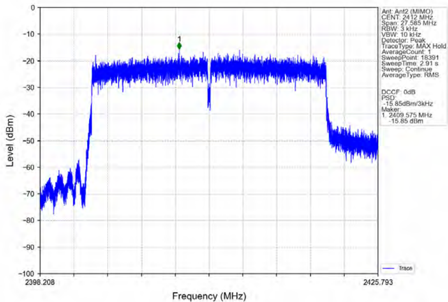
802.11ax(HEW20)_LCH_2412MHz_RU242_Left_Ant2 (MIMO)_NTNV
