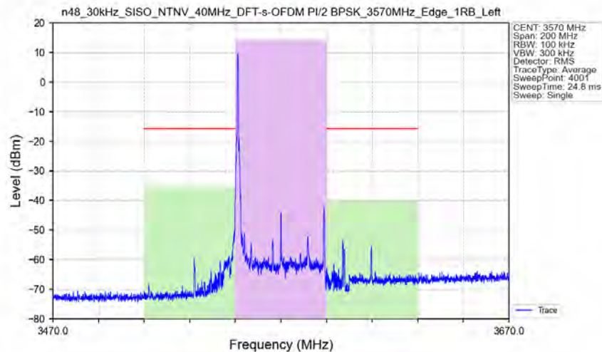
n48_30kHz_SISO_NTNV_40MHz_DFT-s-OFDM PI/2 BPSK_3570MHz_Edge_1RB_Left_Ant1
