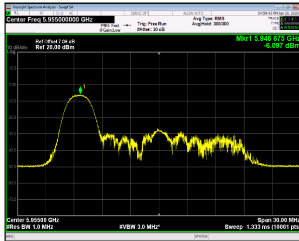
PSD ax20 26@0 5955MHz
