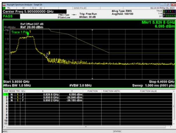
802.11ac20Right Side
