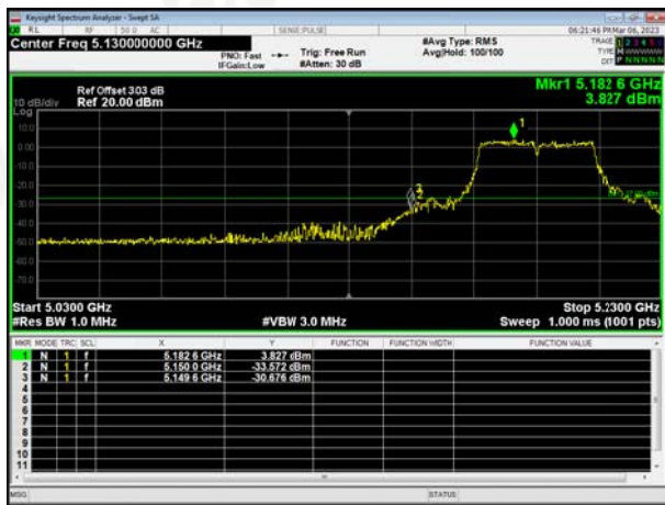
802.11ac40Left Side
