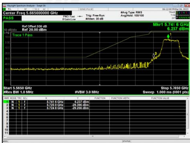
802.11ac20Right Side
