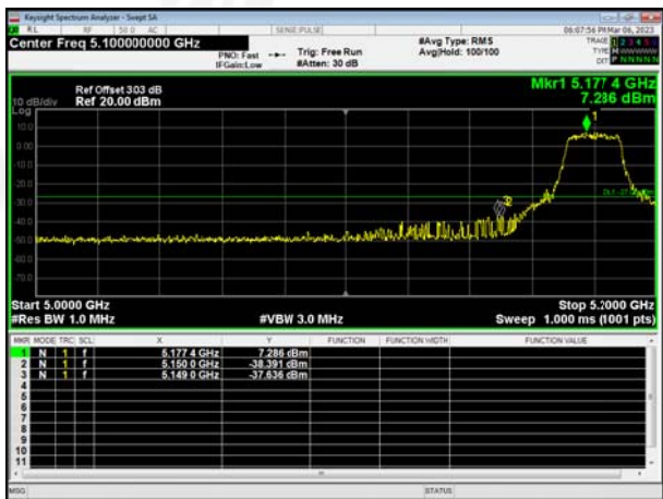
802.11ac20Left Side
