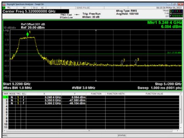
802.11ac20Left Side
