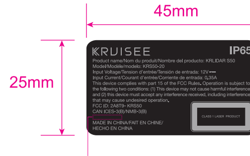
KRS50-20主机认证铭牌警告语标贴
