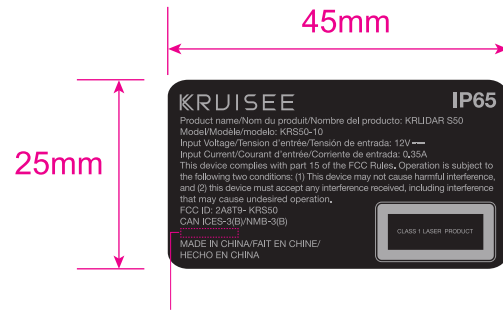
KRS50-10 认证铭牌
