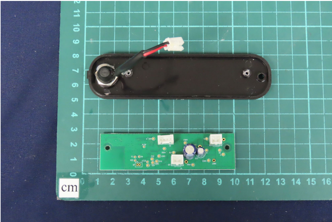
(13) EUT Photo
