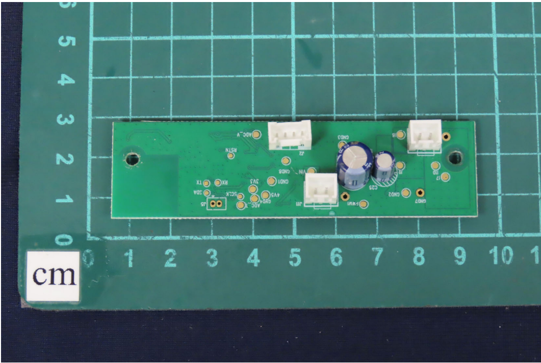
(14) EUT Photo
