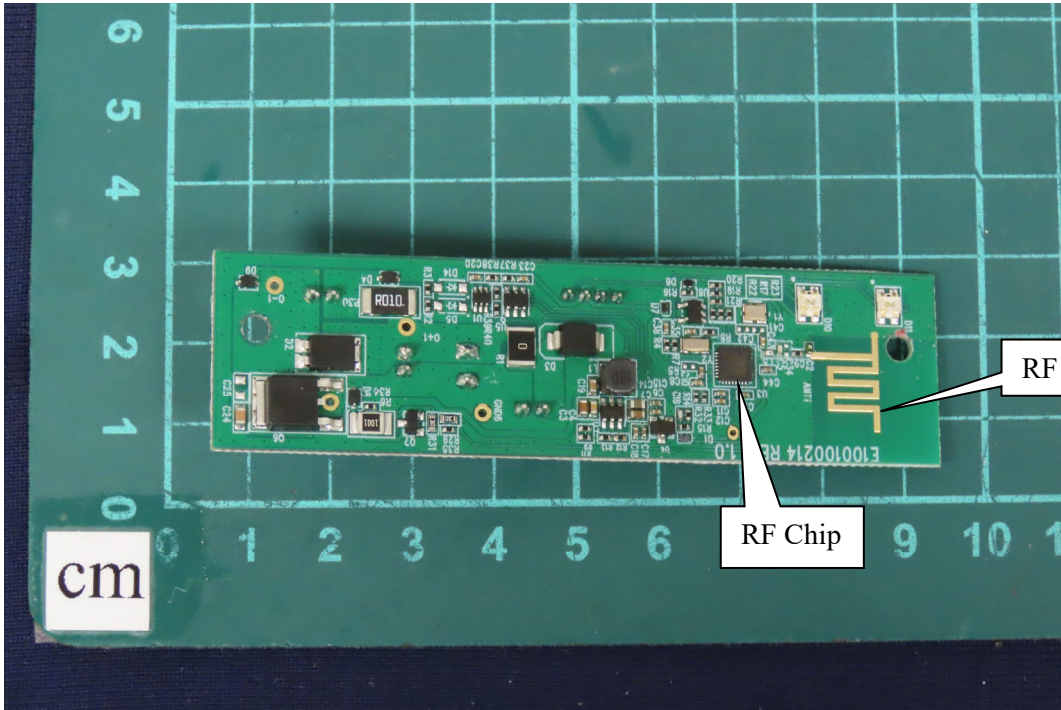
(15) EUT Photo
