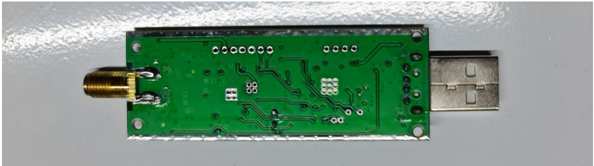
PCB BOTTOM
