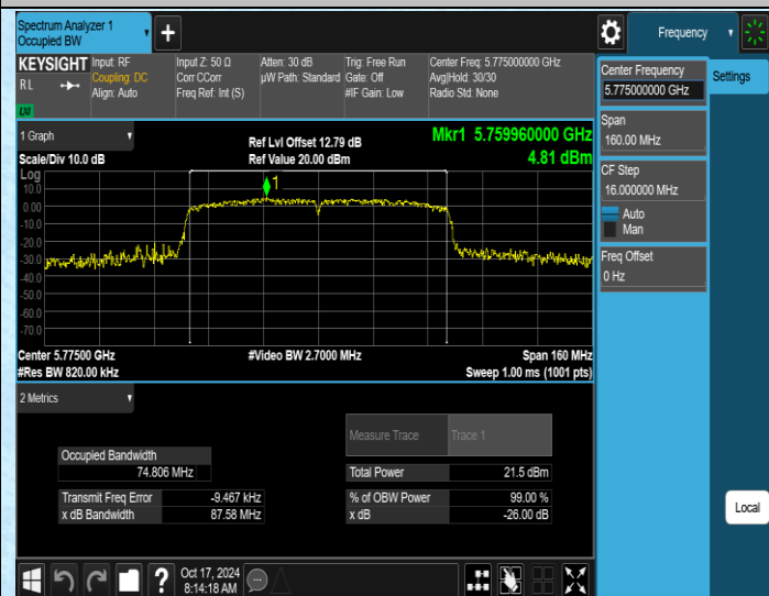
11AC80SISO-Ant2-5775
