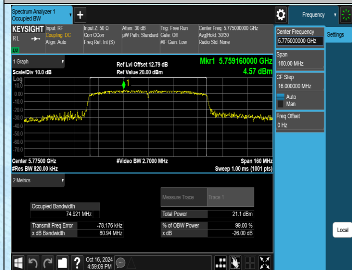
11AC80SISO-Ant1-5775
