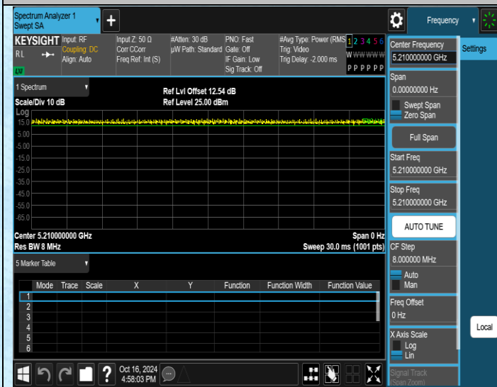
NTNV-11AC80SISO-Ant1-5210
