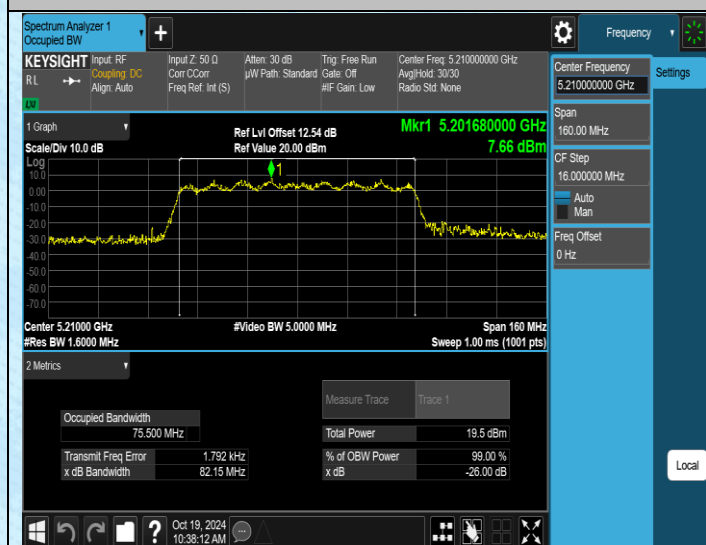
11AC80SISO-Ant3-5210
