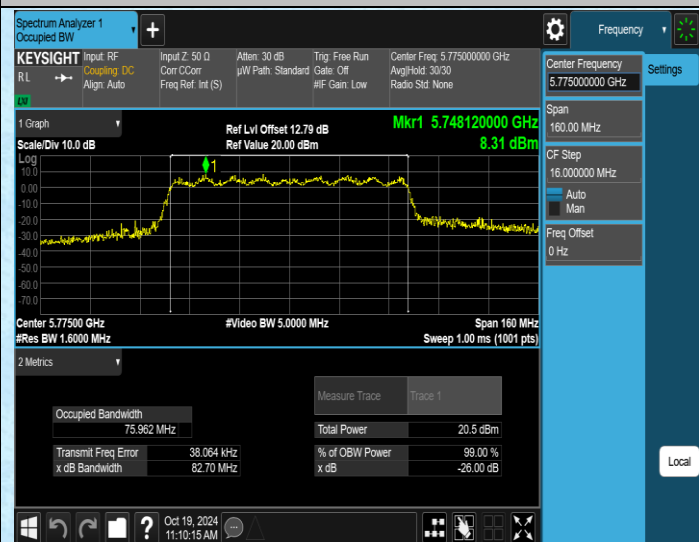
11AC80SISO-Ant4-5775
