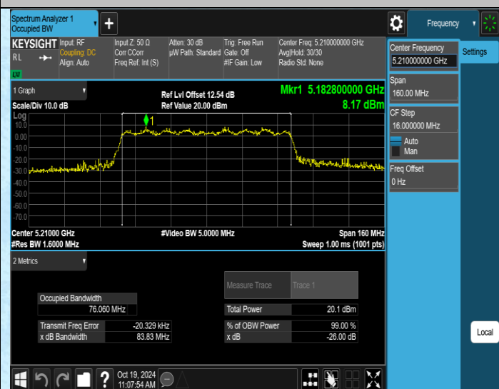
11AC80SISO-Ant4-5210
