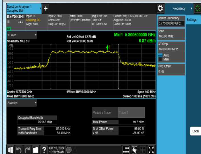
11AC80SISO-Ant3-5775
