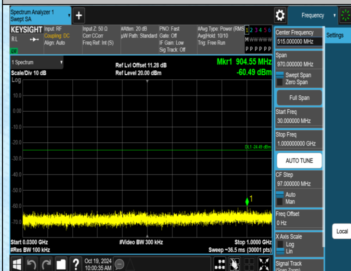
11N20MIMO-Ant4-2412-30~1000-PASS
