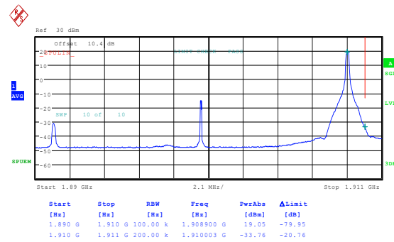
Band2 20MHz 16QAM 19100 1RB#0
