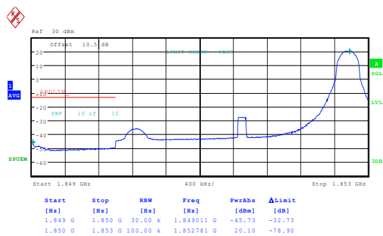
Band2_3MHz_QPSK_18615_1RB#0
