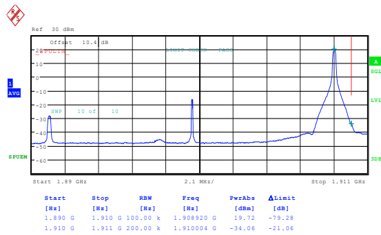
Band2 20MHz QPSK 19100 1RB#0
