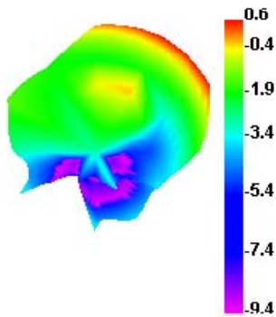
5150.000MHz E1
