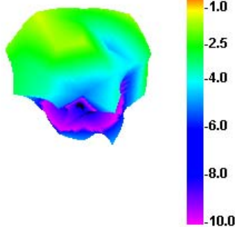
5850.000MHz E1
