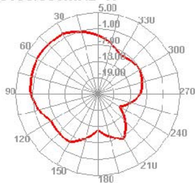
5150.000MHz H
