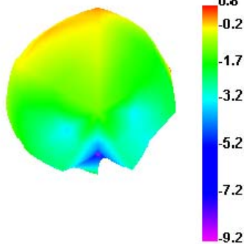
5500.000MHz E1
