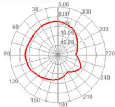
2500.000MHz E2
