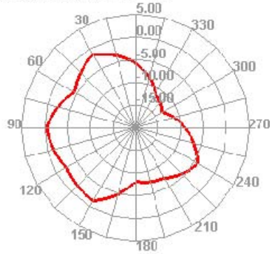
5150.000MHz E2
