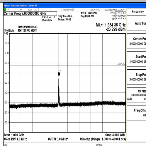
Band2 1.4MHz QPSK 18607 1RB#0 1000~3000 1000~3000
