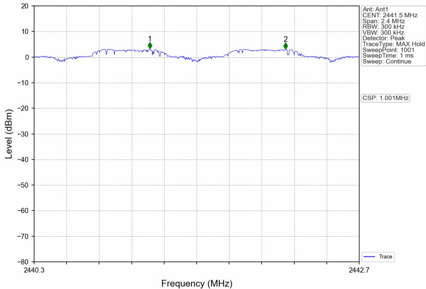
Pi/4DQPSK_2DH5_HOPP_Ant1_NTNV
